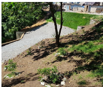
Рисунок 44. Проведение противооползневых мероприятий в месте пересечения р. Котловки и Севастопольского проспекта (2019 год)
