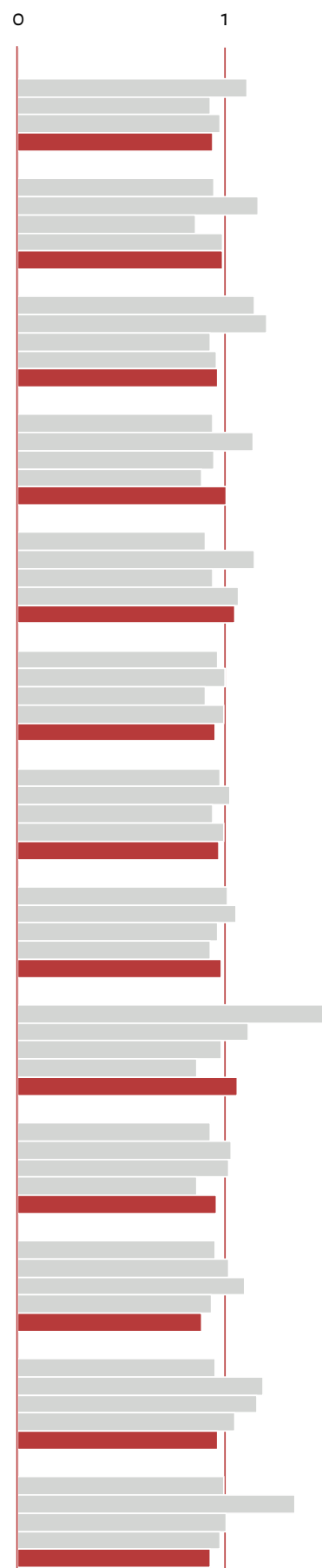
Рисунок 12. БПК 5 в створах Москвы-реки
