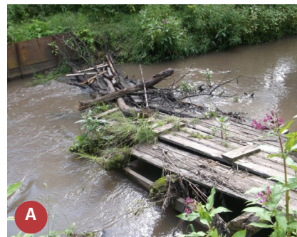
Рисунок 34. Участок русла р.Сходня А. перекрытие русла разрушенным мостом, Б. участок перекрытого русла после расчистки
