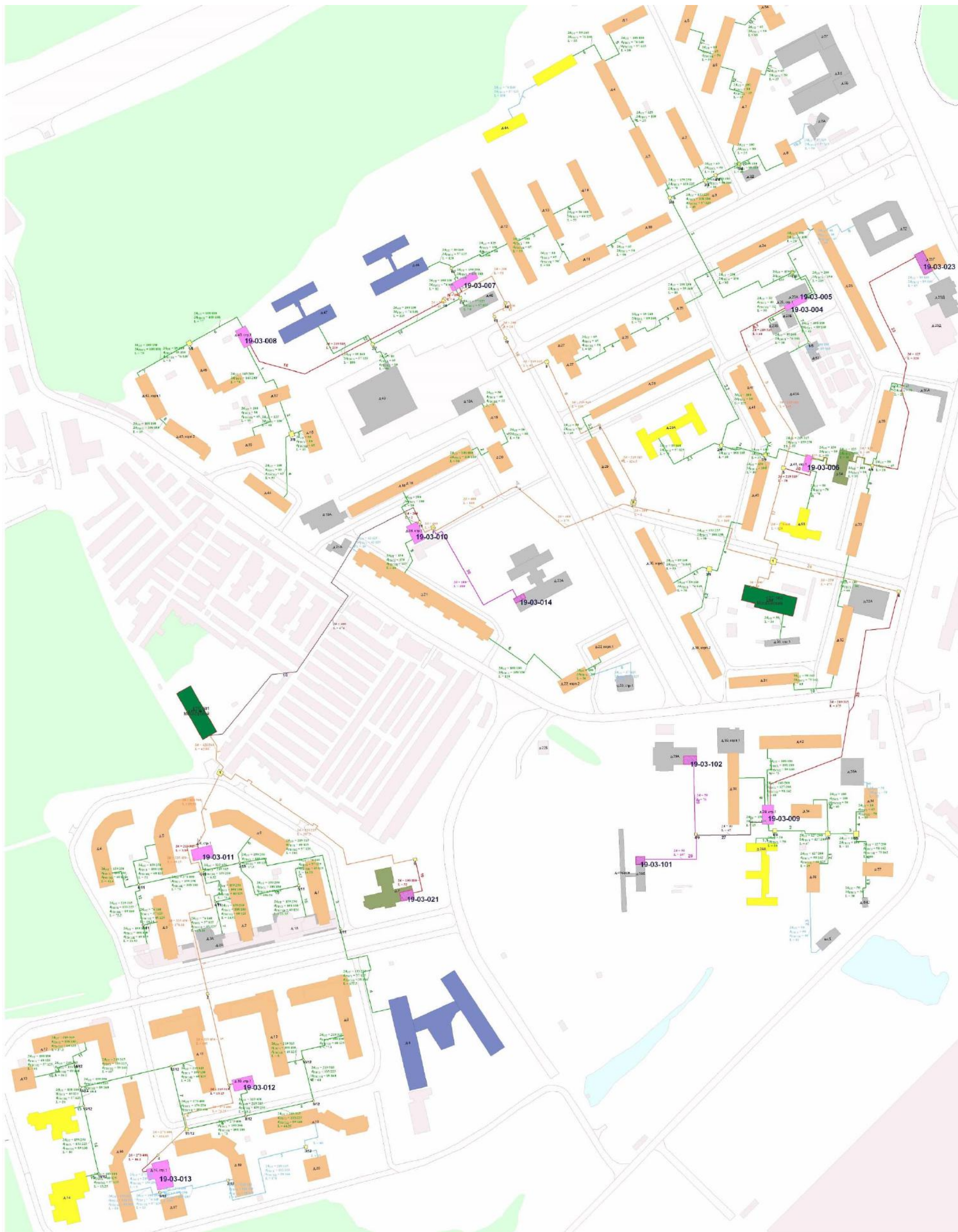
Рисунок В.2.8 - Схема тепловых сетей от КТС-1 «Московский» и КТС-2 «Московский»
