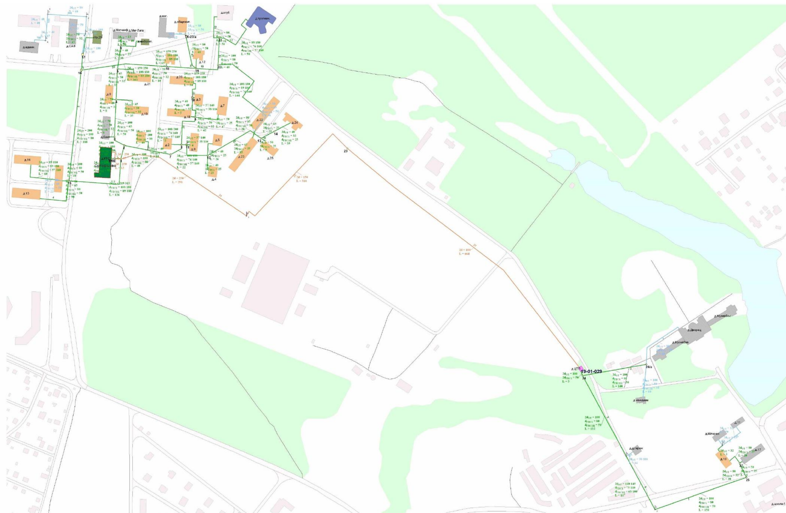
Рисунок В.2.2 - Схема тепловых сетей от КТС «Остафьево»
