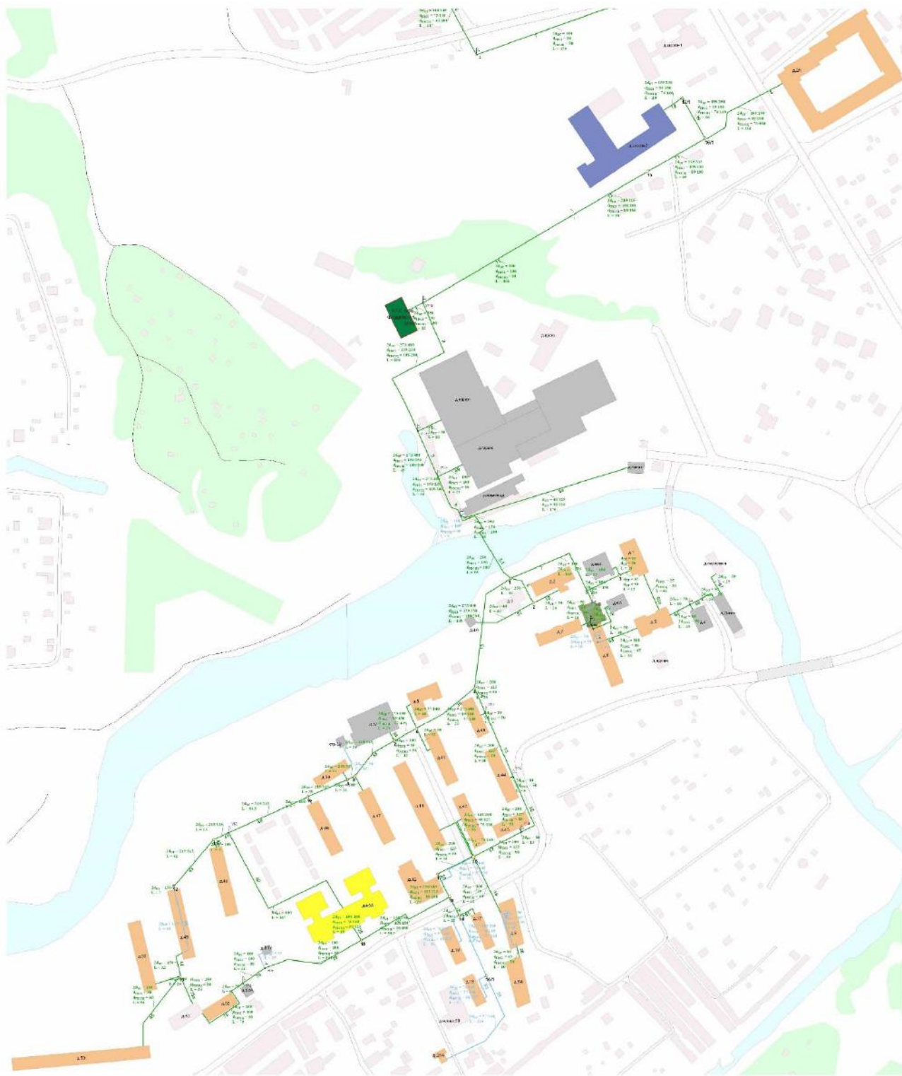
Рисунок В.2.3 - Схема тепловых сетей от КТС «Фабрика им. 1 Мая»
