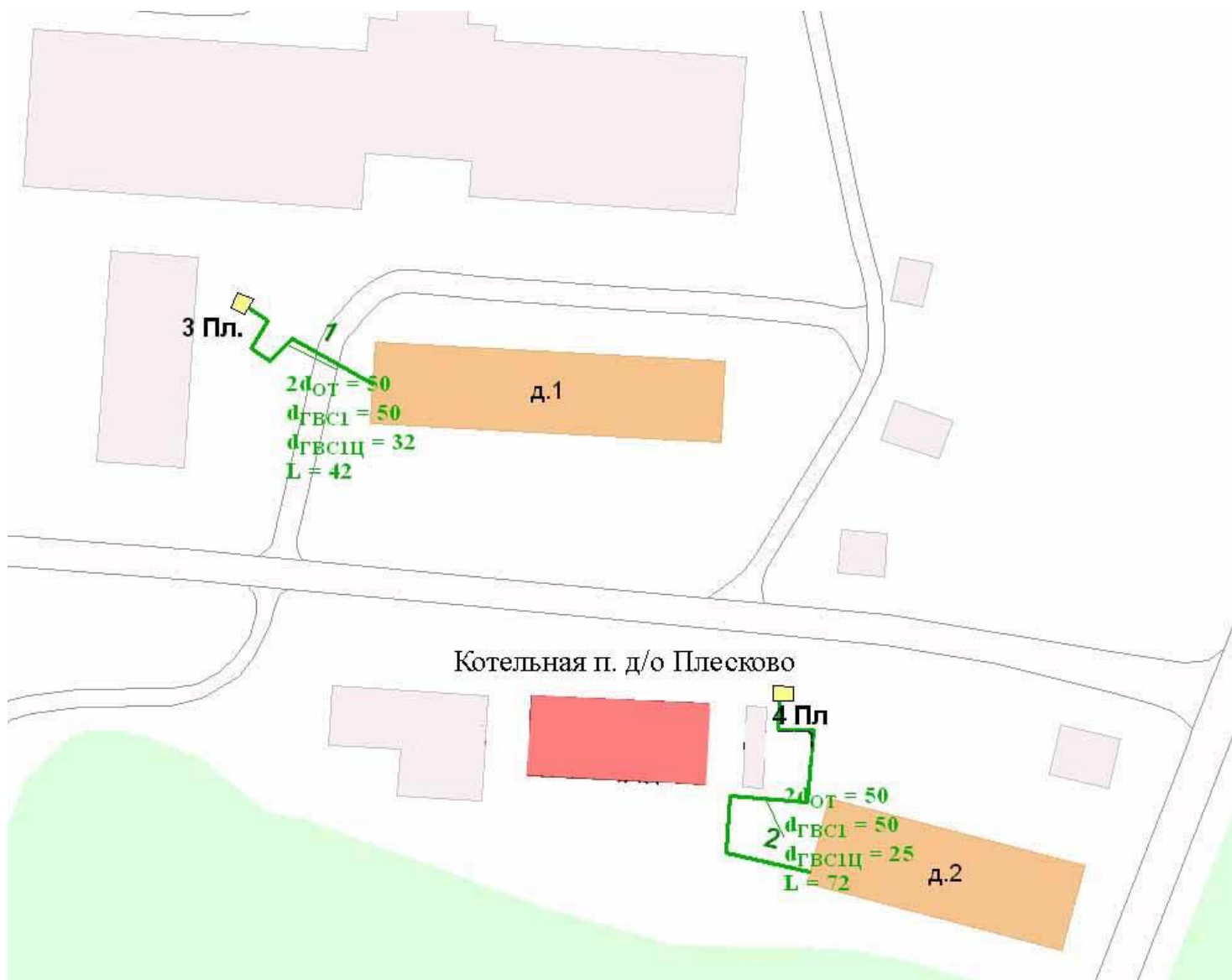
Рисунок В.3.2 - Схема тепловых сетей от котельной п. д/о Плесково
