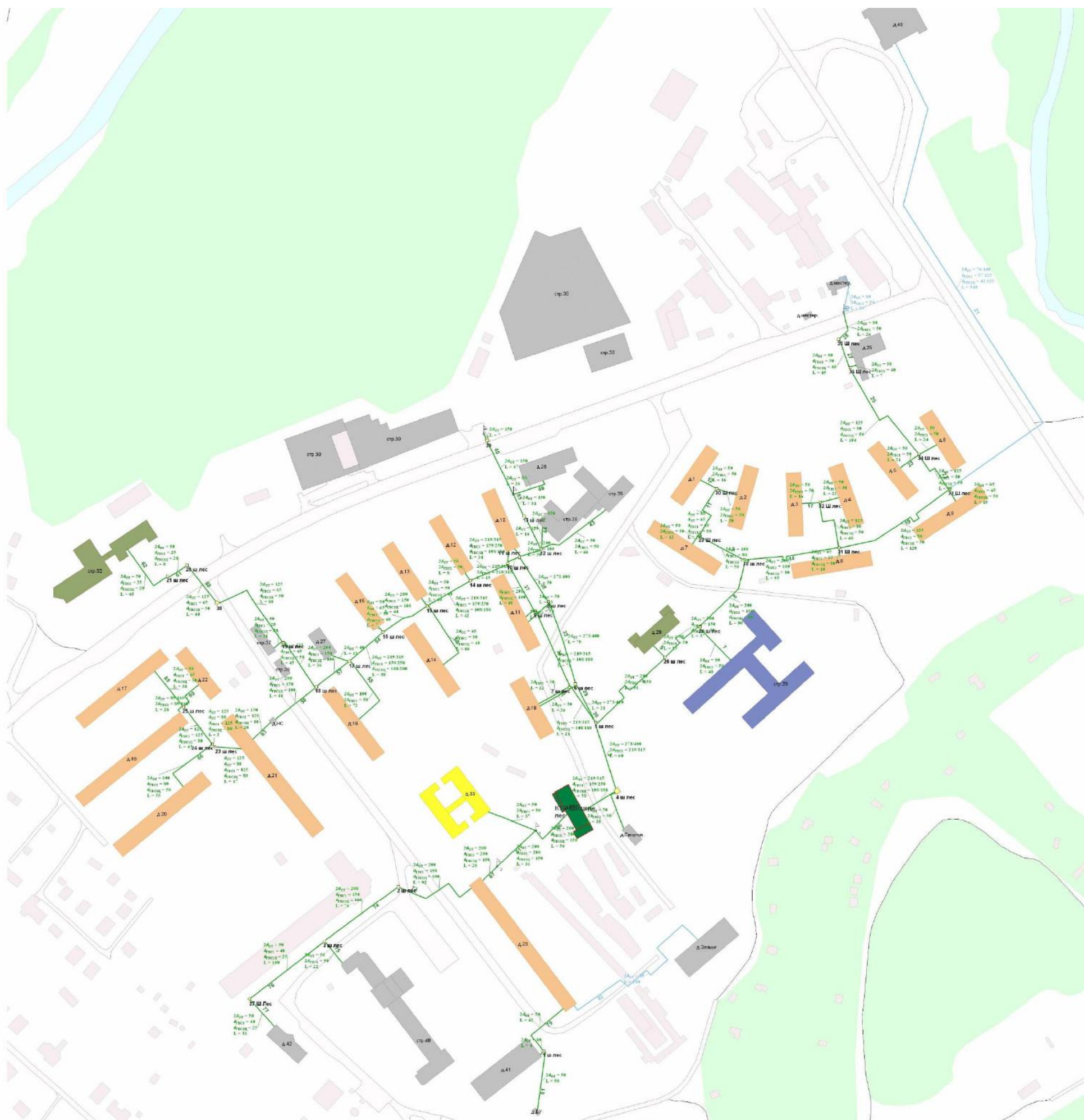
Рисунок В.2.18 - Схема тепловых сетей от КТС «Шишкин Лес»
