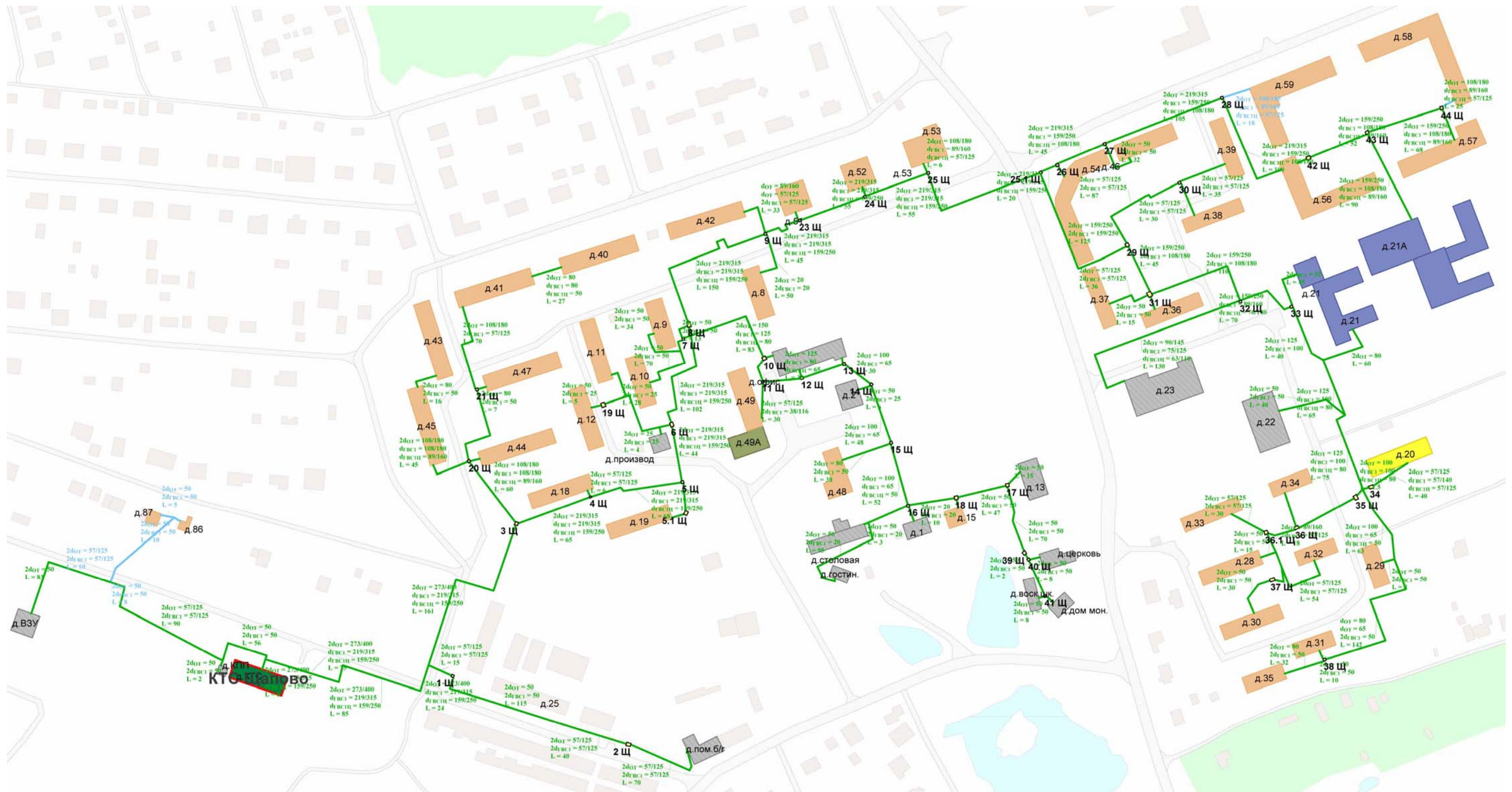
Рисунок В.2.20 - Схема тепловых сетей от КТС «Щапово»
