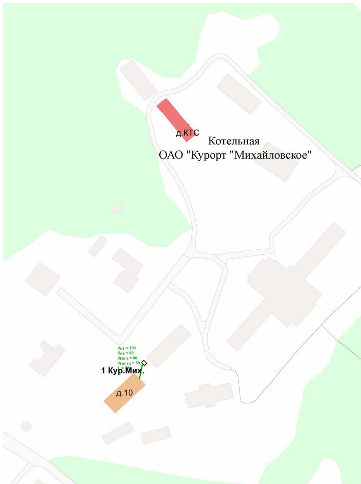
Рисунок В.3.3 - Схема тепловых сетей от котельной ОАО «Курорт «Михайловское»
