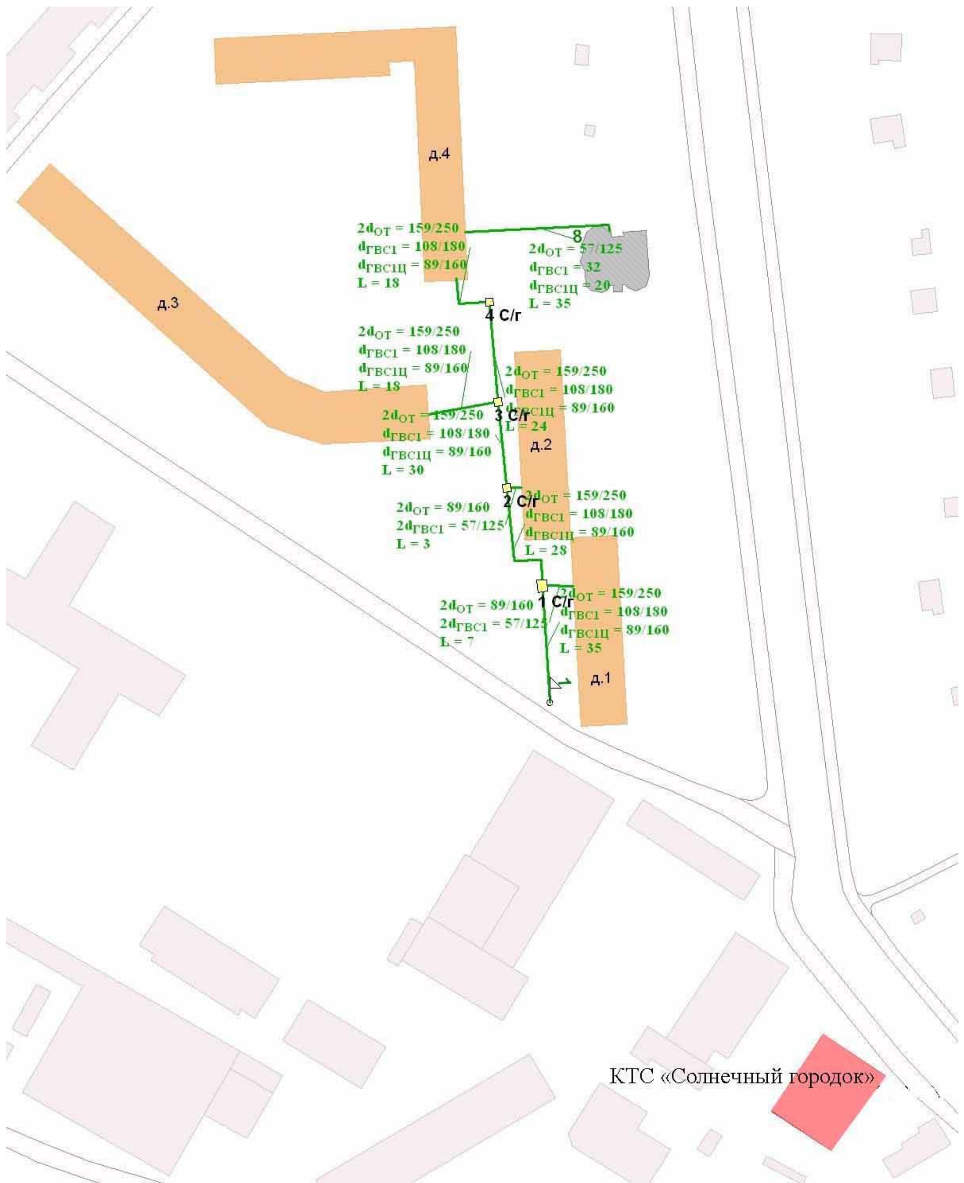
Рисунок В.3.4 - Схема тепловых сетей от котельной КТС «Солнечный городок»
