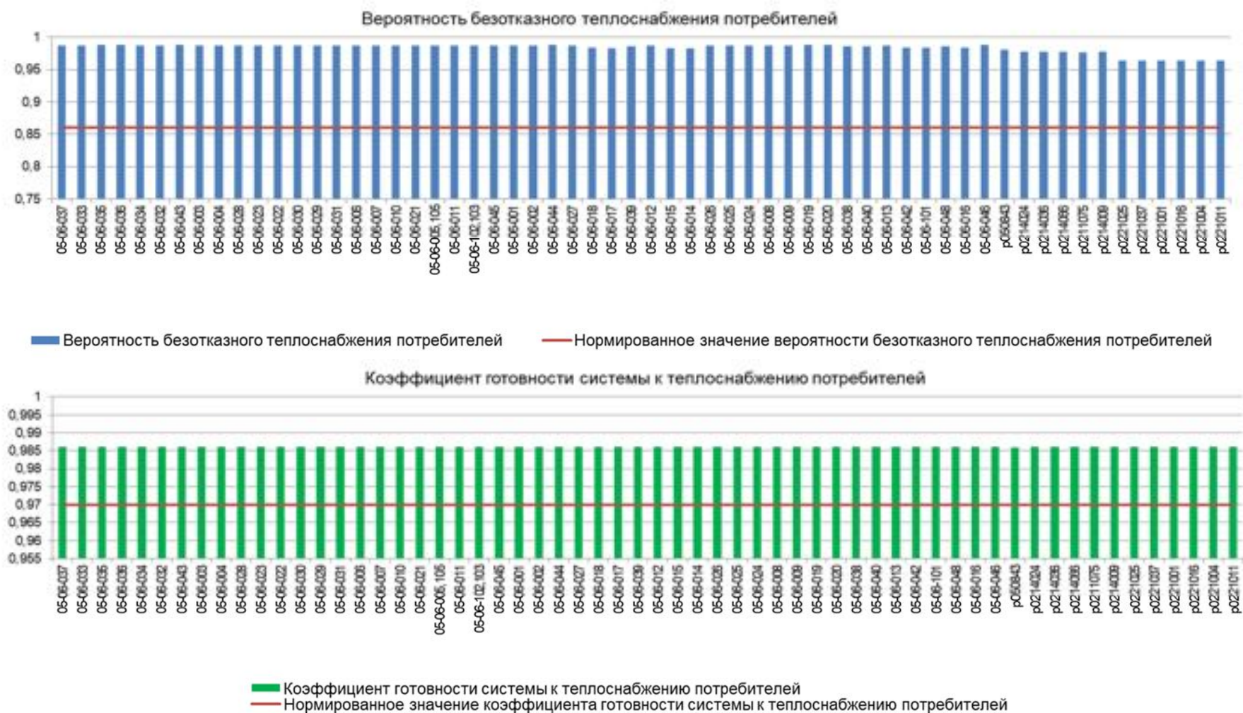
Рисунок А.9 – Вероятность безотказного теплоснабжения и коэффициент готовности системы к теплоснабжению потребителей ТЭЦ-22
