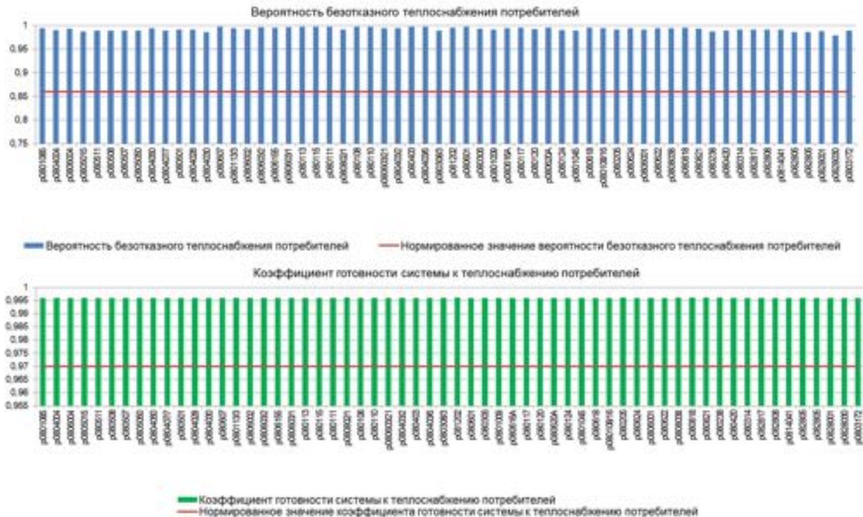
Рисунок А.7 – Вероятность безотказного теплоснабжения и коэффициент готовности системы к теплоснабжению потребителей ТЭЦ-20
