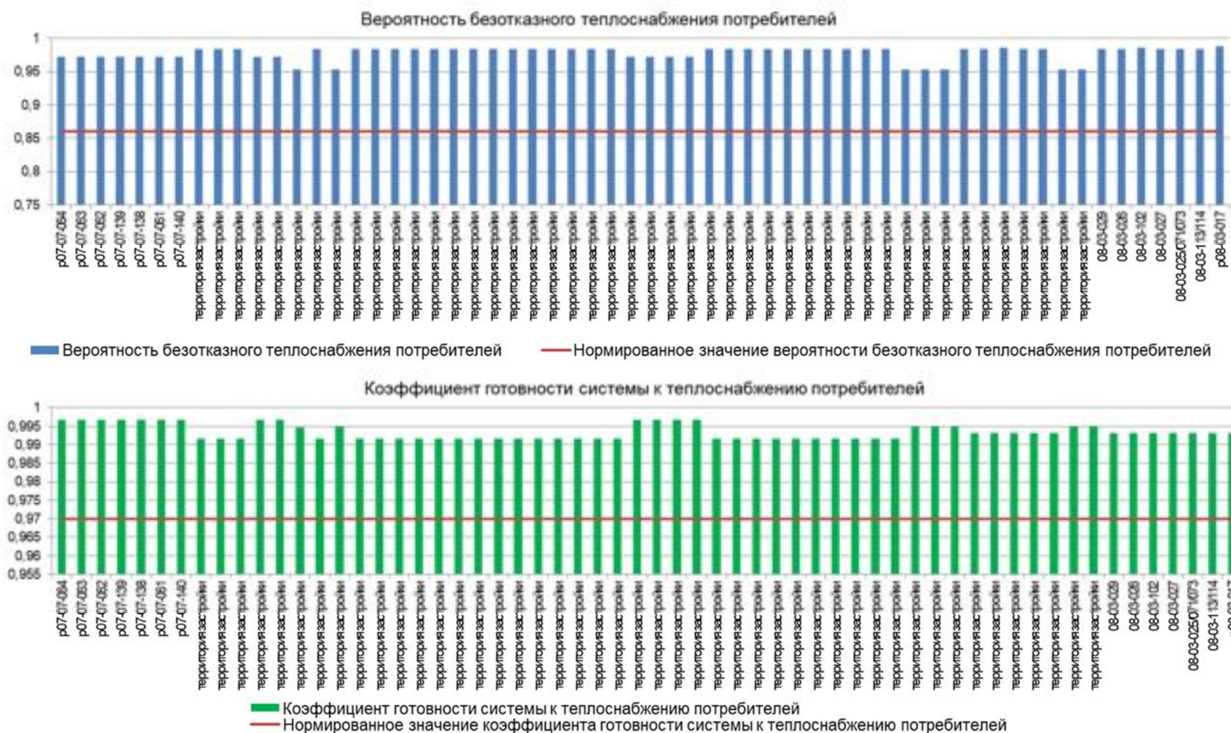
Рисунок А.11 – Вероятность безотказного теплоснабжения и коэффициент готовности системы к теплоснабжению потребителей ТЭЦ-25
