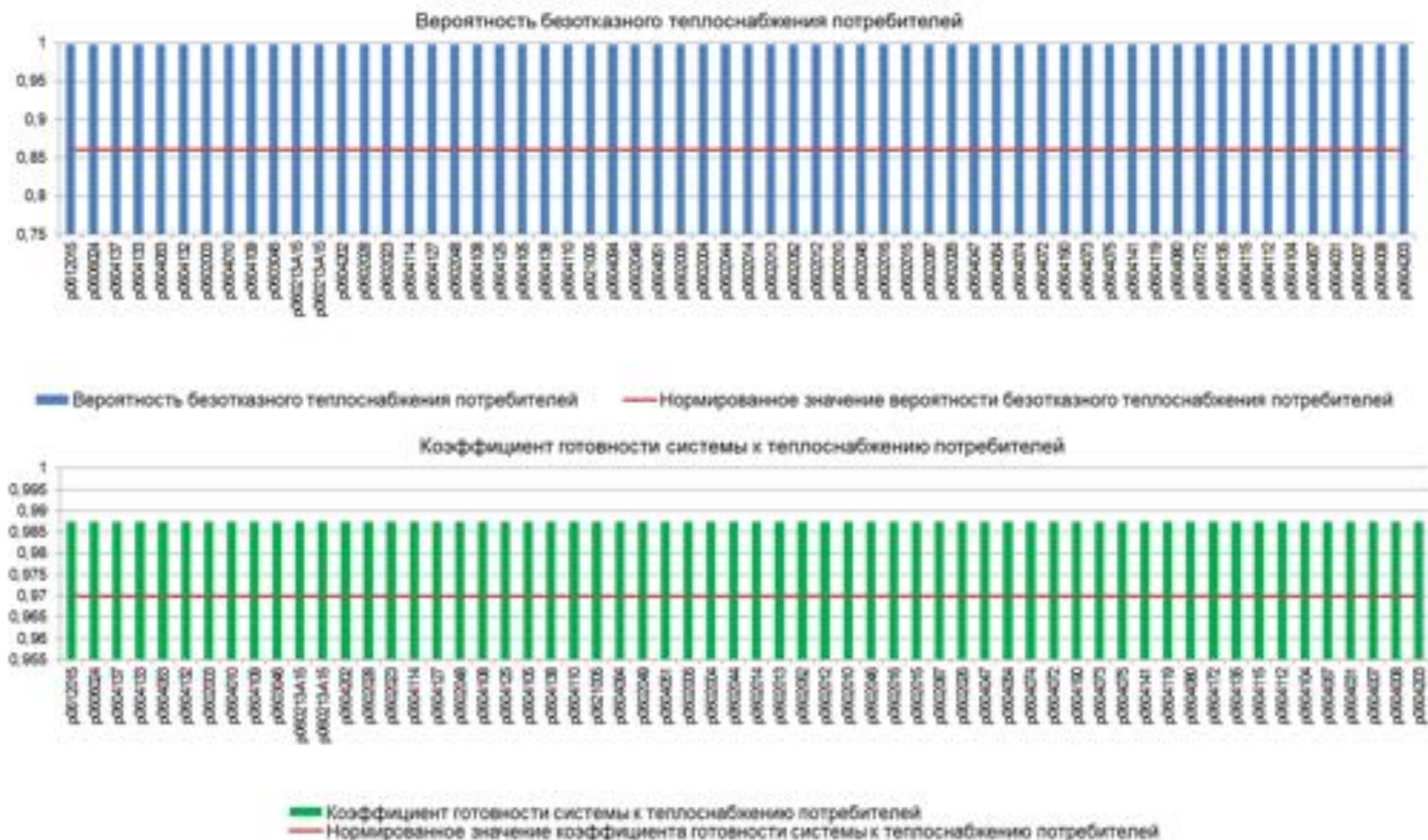
Рисунок А.10 – Вероятность безотказного теплоснабжения и коэффициент готовности системы к теплоснабжению потребителей ТЭЦ-23
