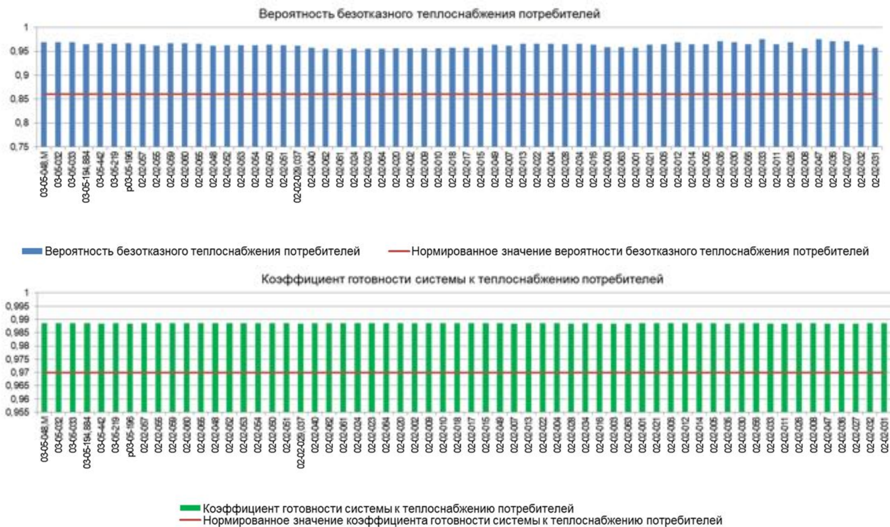
Рисунок А.8 – Вероятность безотказного теплоснабжения и коэффициент готовности системы к теплоснабжению потребителей ТЭЦ-21
